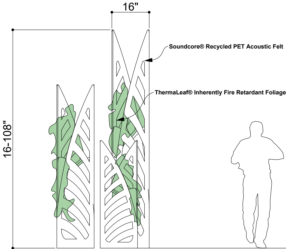
① ELEVATION 1
